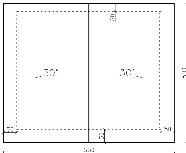
RZUT POŁĄCI DACHOWYCH
