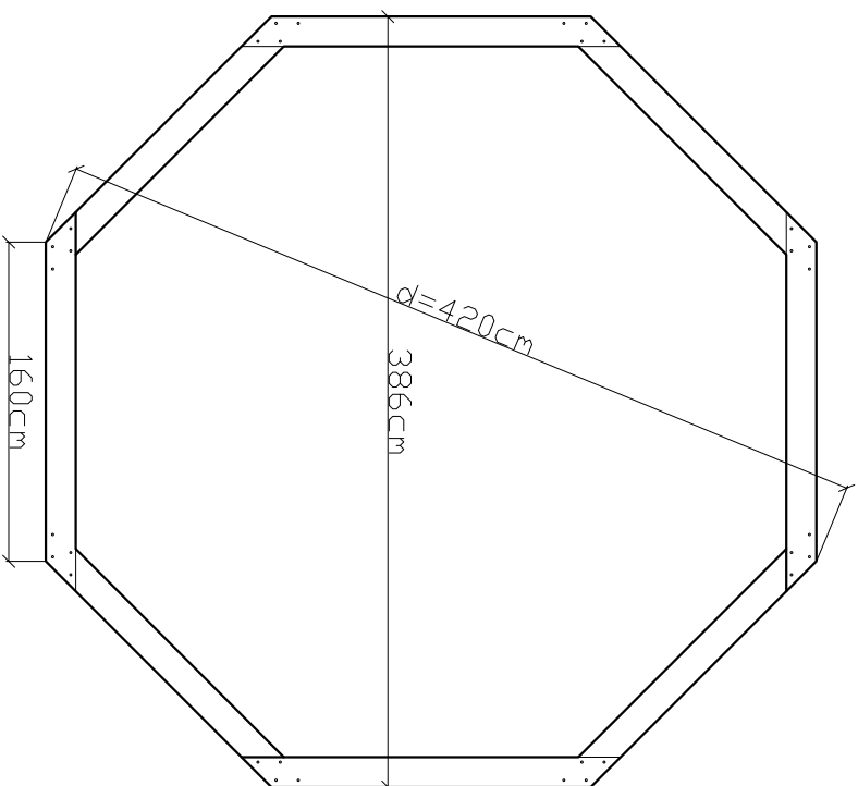
Rzut podsławy
